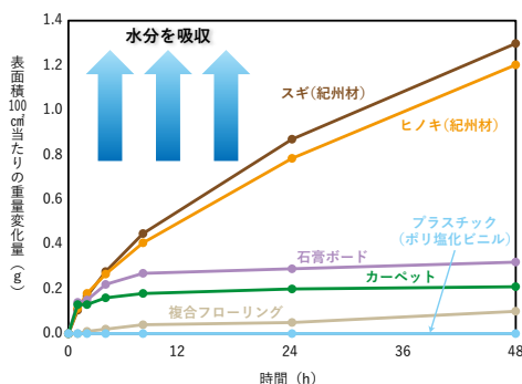
図 高湿度環境(吸湿)に伴う重量変化
