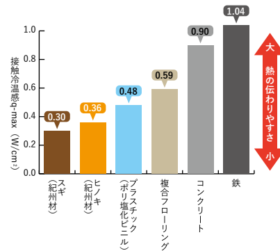
図 各材料の接触冷感
