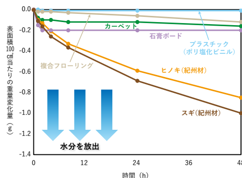
図 低湿度環境(放湿)に伴う重量変化
